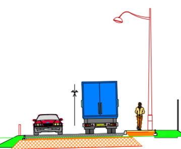
ZA du Val d'Or - Coupe M-M
