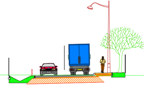
ZA du Val d'Or - Coupe L-L
